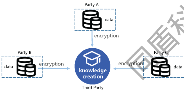
图3. 信息层联邦
